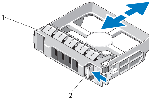
图 3-5. 卸下或安装硬盘驱动器挡片
