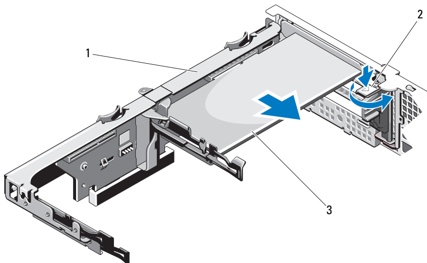
图 3-11. 安装或卸下扩充卡
