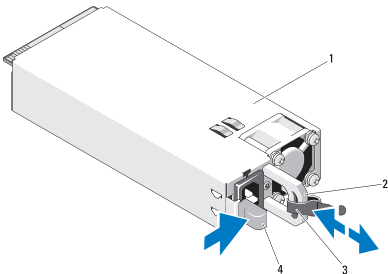
图 3-9. 卸下和安装冗余电源设备
