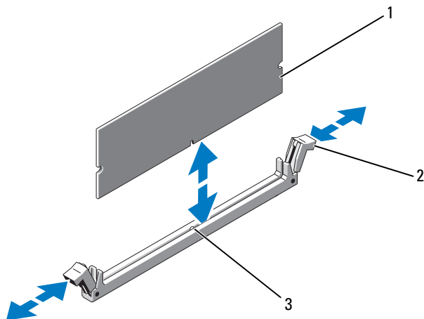
图 3-10. 安装和卸下内存模块
