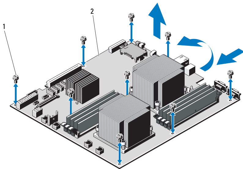
图 3-22. 卸下和安装系统板
