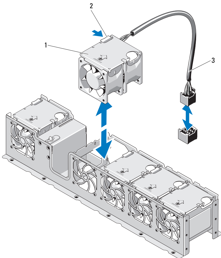
图 3-8. 卸下和装回风扇
