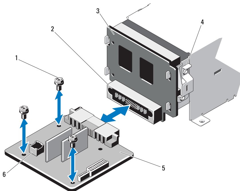
图 3-21. 卸下和装回配电板
