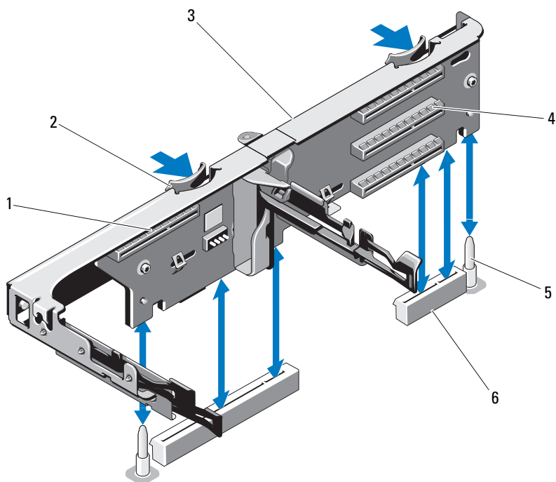
图 3-12. 安装或卸下扩充卡提升板
