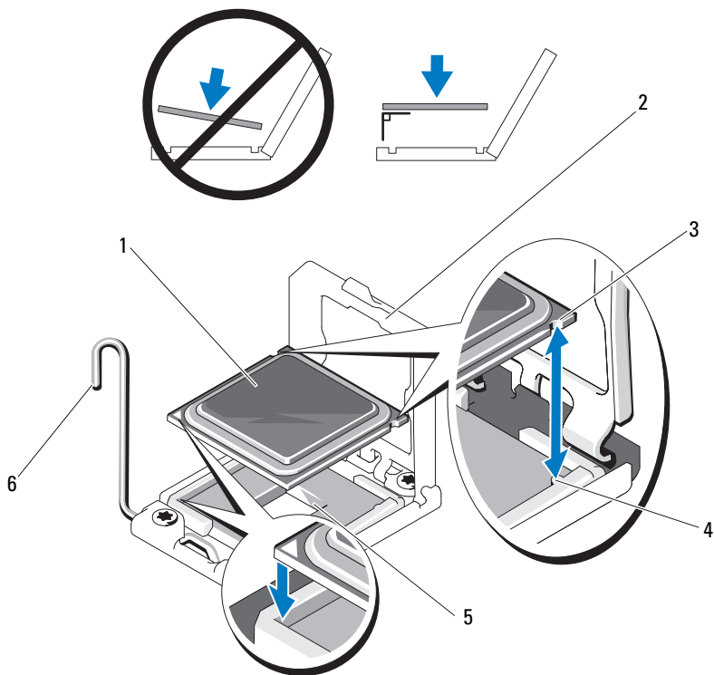
图 3-17. 安装和卸下处理器
