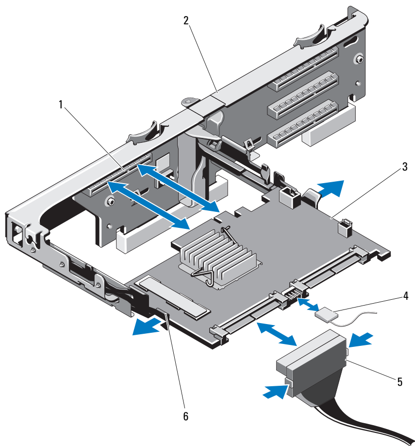
图 3-13. 安装和卸下存储控制器卡
