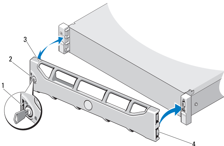
图 3-2. 卸下和装回前挡板
