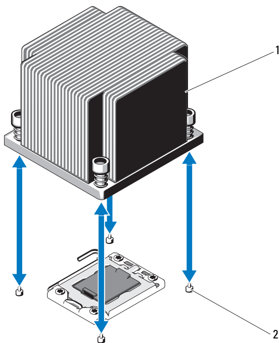
图 3-16. 安装和卸下散热器
