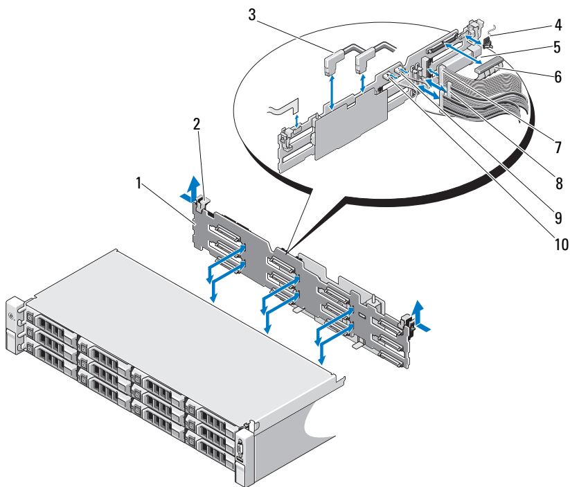
图 3-20. 卸下和安装 SAS 背板
