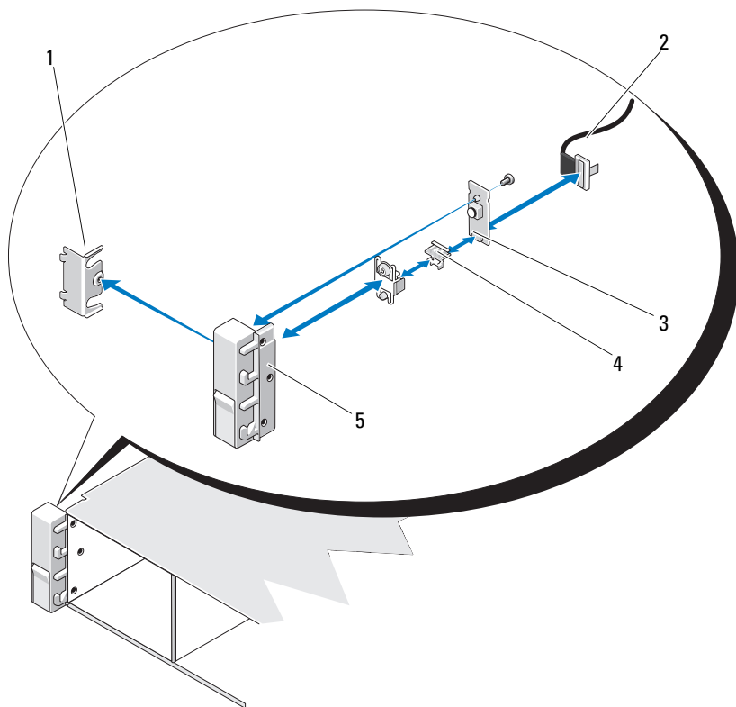
图 3-19. 卸下和安装控制面板—LED（具有 12 个硬盘驱动器的系统）
