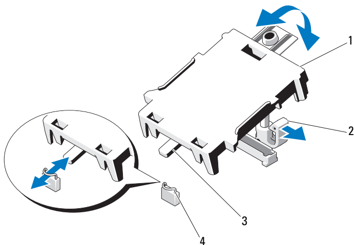
图 3-14. 安装或卸下 iDRAC6 Express 卡
